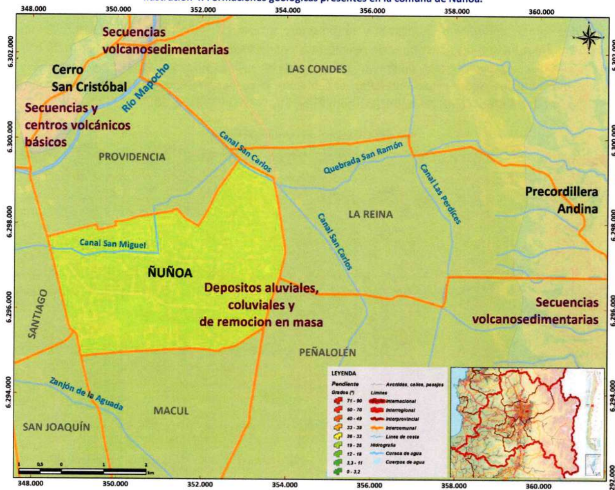
Ilustración 4. Formaciones geológicas presentes en la comuna de Nuñoa.
