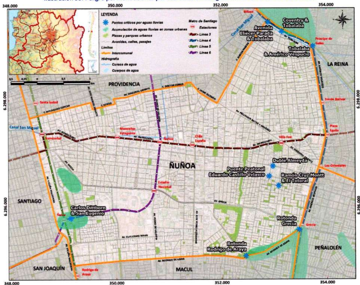
Ilustración 53. Peligro por inundaciones por acumulación de aguas lluvias en la comuna de Nuñoa.
