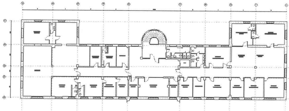
PLANTA EXISTENTE
