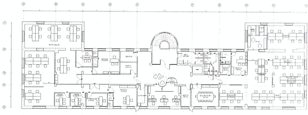
PLANTA ARQUITECTURA
